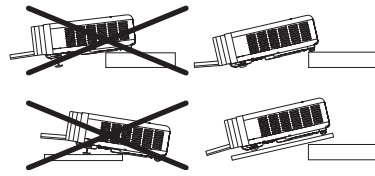
<Richtiges Aufstellen des Projektors>
